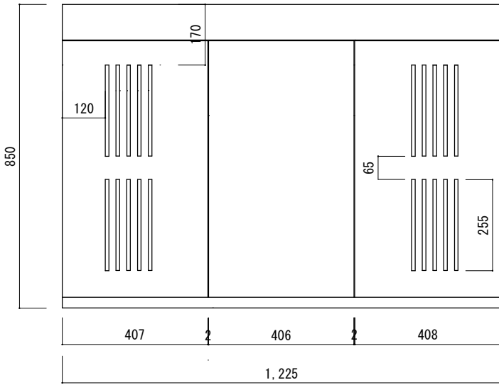
水槽台正面図
