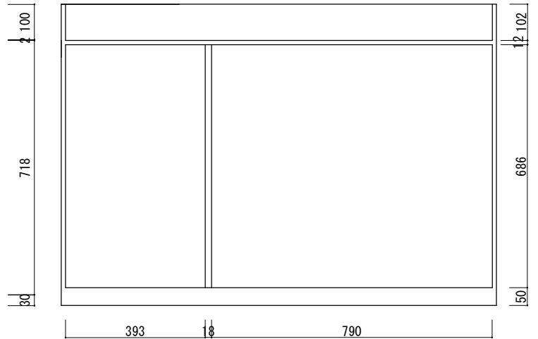
水槽台内寸図
