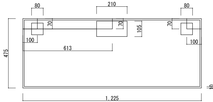
水槽台上面図(開口寸法)
