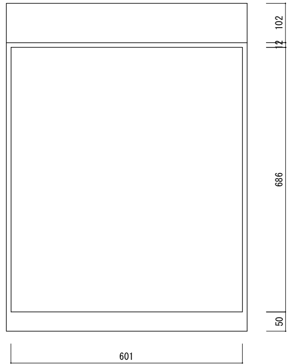
水槽台内寸図
