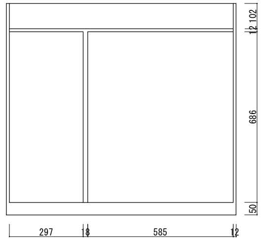
水槽台内寸図
